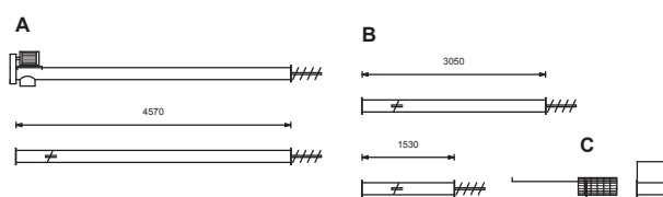
Ruuvikuljetin toimitetaan kasaamattomana.
