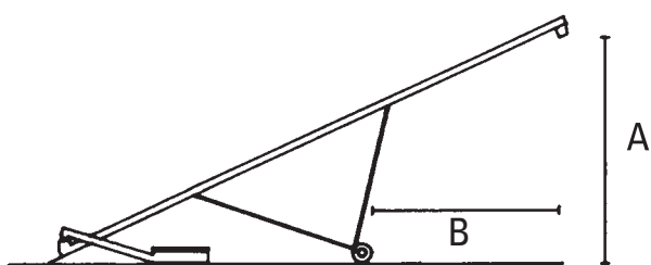
Målskitse for MK rørsnegle ▼
